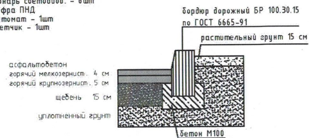
Разрез дороги 1-1
