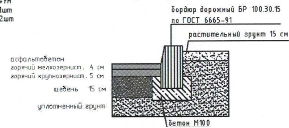
Разрез дороги 1-1
