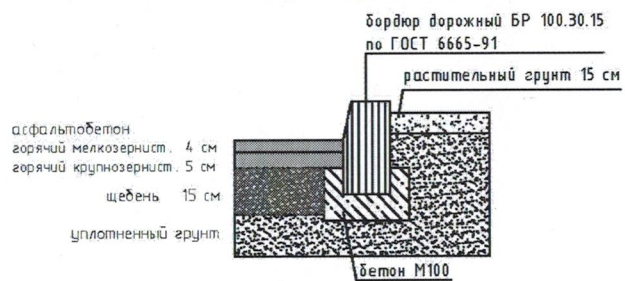
Разрез дороги 1-1
